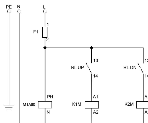
۳. نقشه مدار فرمان با دو عدد کنتاکتور
