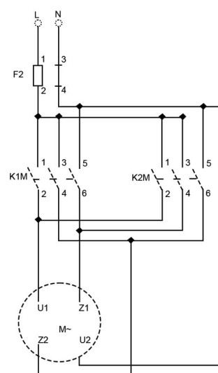
۱. نقشه مدار قدرت چپ گرد راست گرد تک فاز
